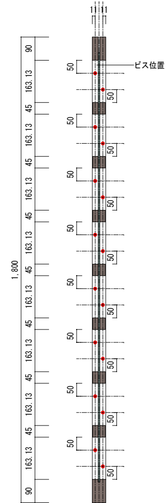
姿図
