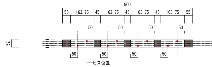
平面図 (上部框)
