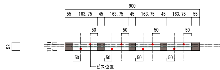
平面図 (下部框)
