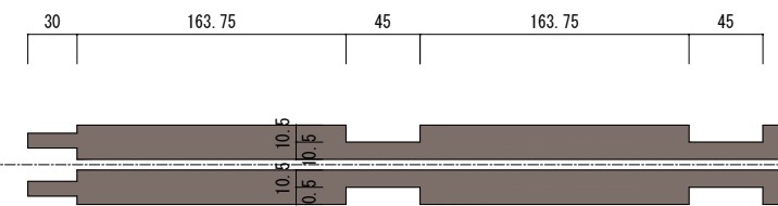
横椽平面
