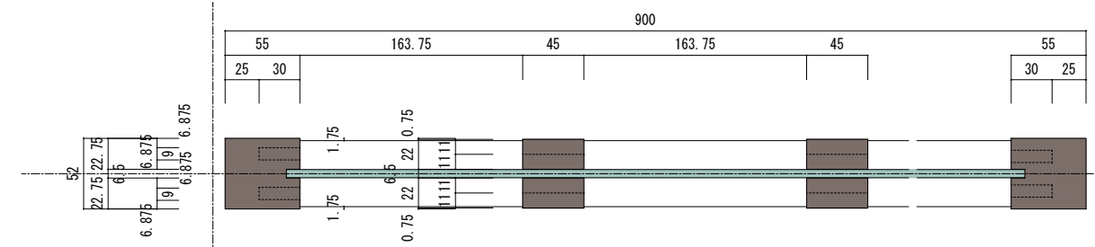
縦椽平面
